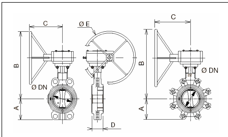
Рис. 2 Габаритные размеры APORIA – RM
