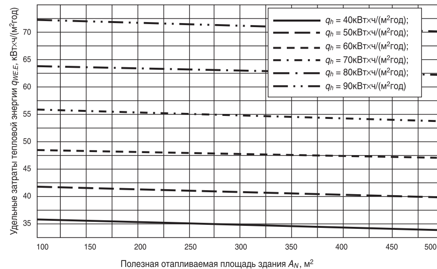
Рис. 14. Зависимость тепловых затрат здания от теплотери и отапливаемой площади
