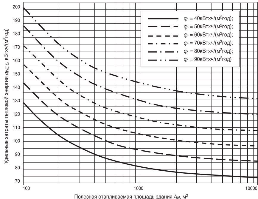
Рис. 8. Зависимость тепловых затрат здания от теплопотерь и отапливаемой площади
