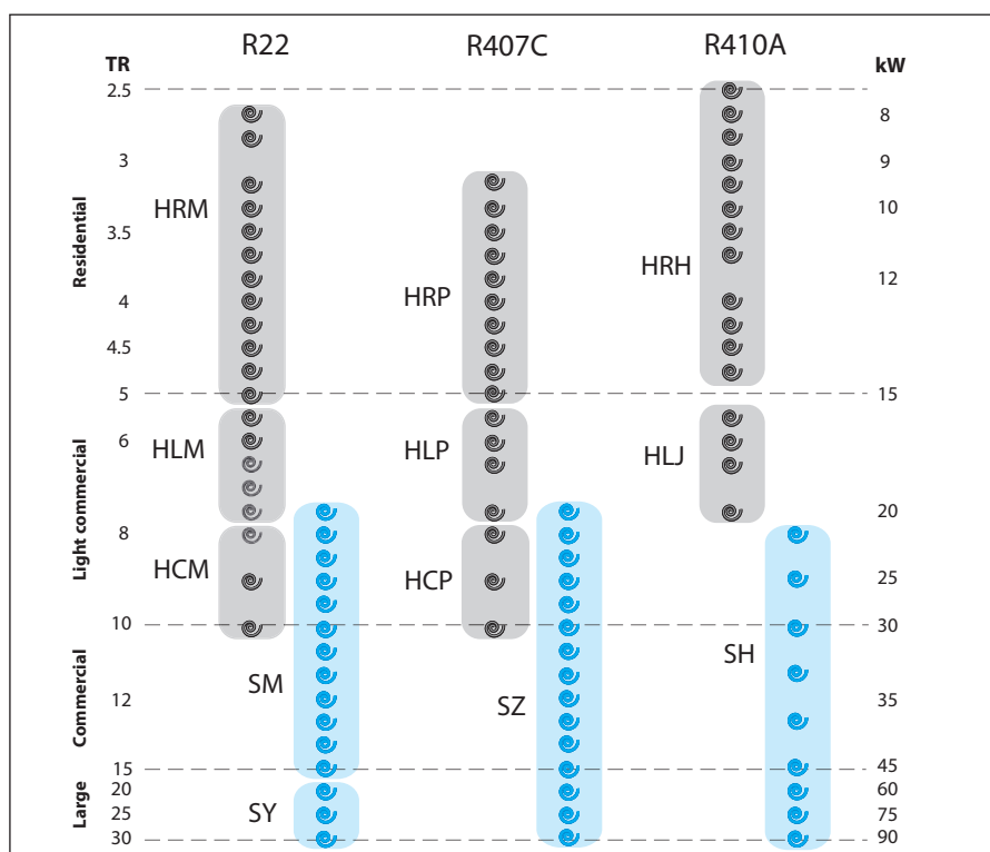
Gamme complète de compresseurs Danfoss Scroll
