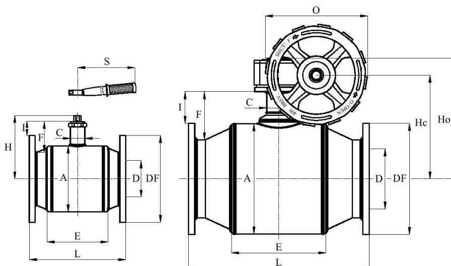
Рис. 2. Габаритные и присоединительные размеры шаровых кранов JiP, фланцевые.
