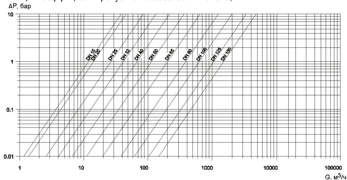
Рис. 3. Диаграмма выбора шарового крана JiP.
