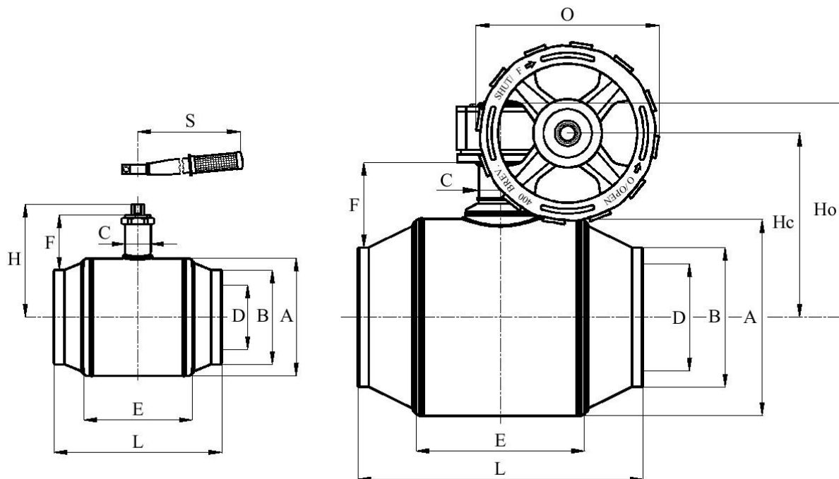
Рис. 1. Габаритные и присоединительные размеры шаровых кранов JiP с патрубками под приварку.
